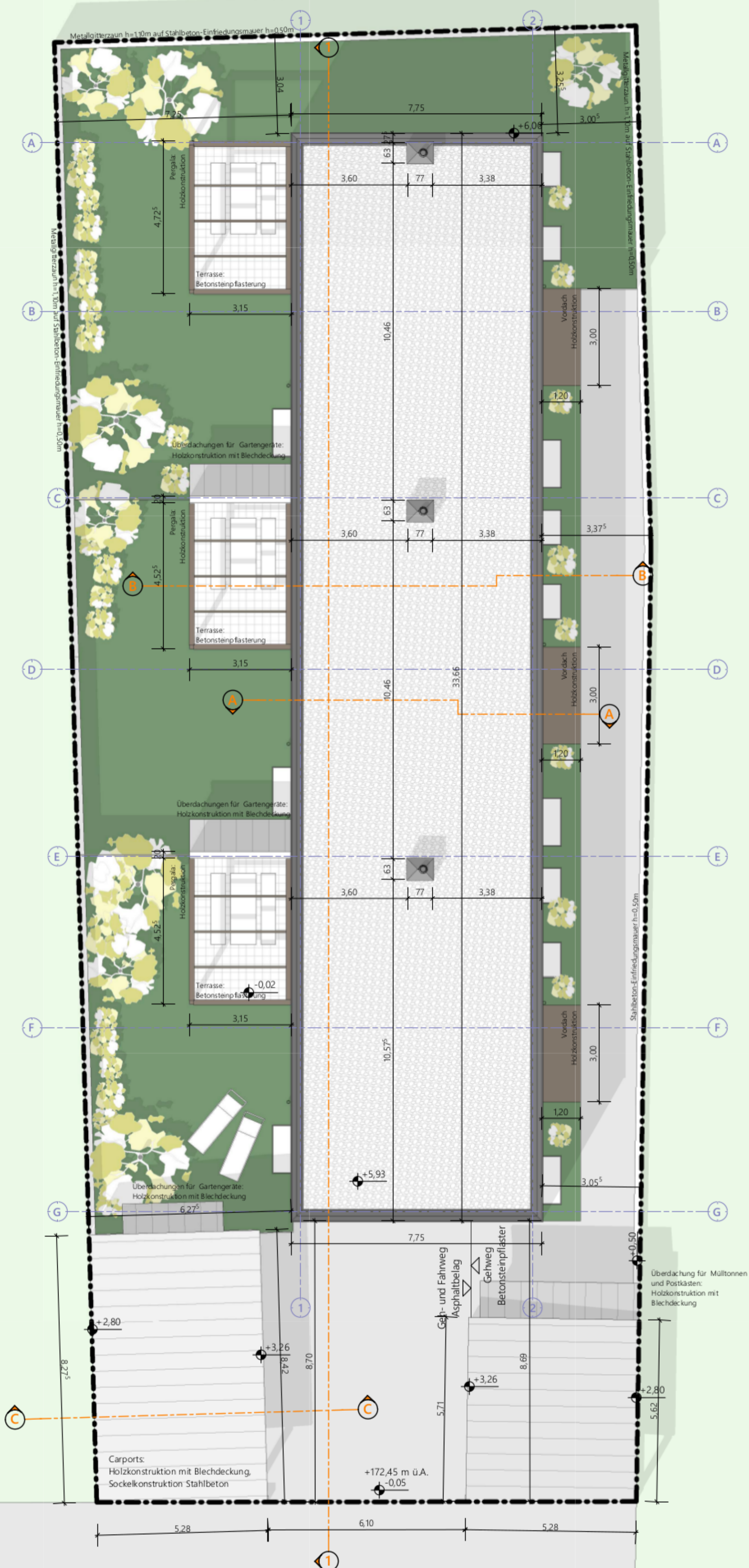
Dachdraufsicht M 1 : 100
